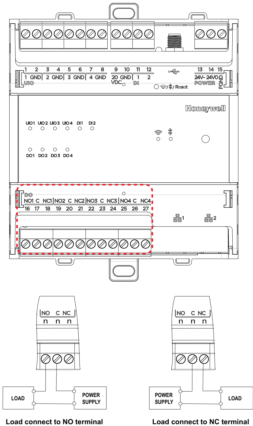
Fig. 9. Digital/Relay Outputs
