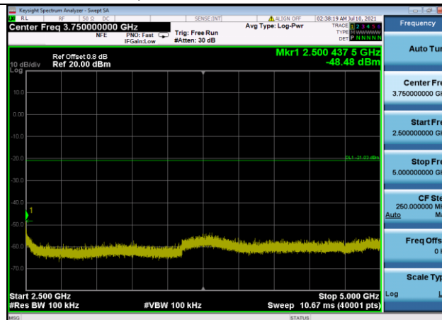
802.11n(HT40),2452MHz,Ant0,Plot 4,2500MHz~5000MHz
