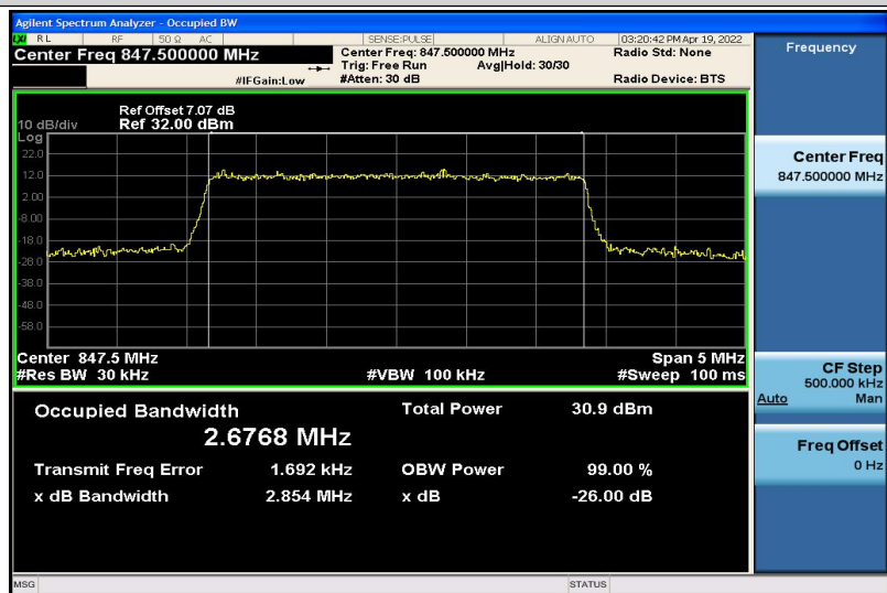
Band5-3MHz-QPSK-20635-15RB#0-2.6768
