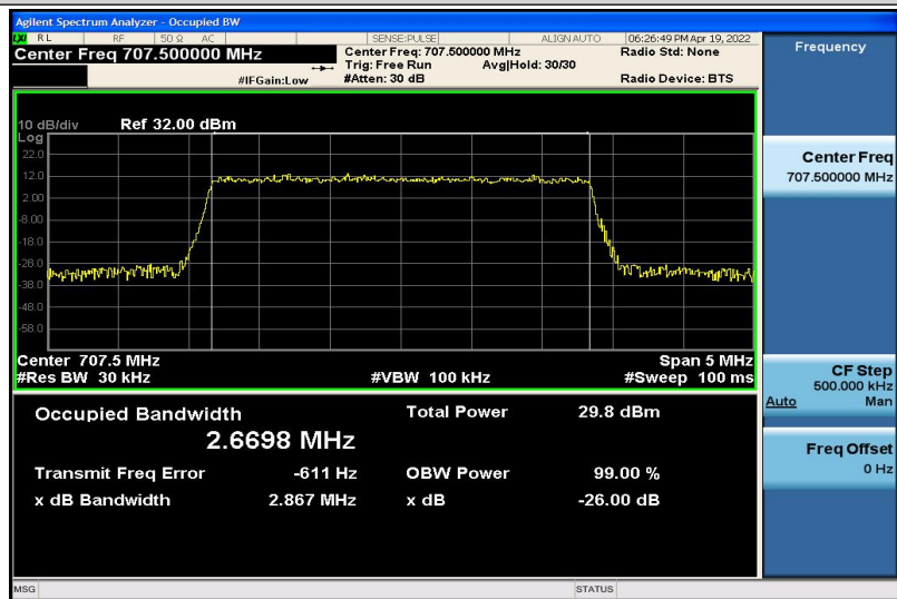
Band12-3MHz-16QAM-23095-15RB#0-2.6698
