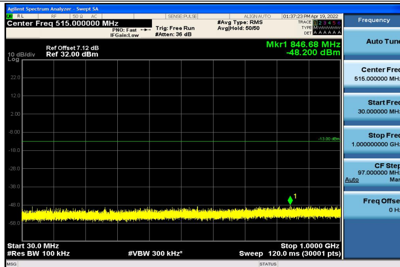
Band4-5MHz-QPSK-20375-1RB#0-30~1000MHz
