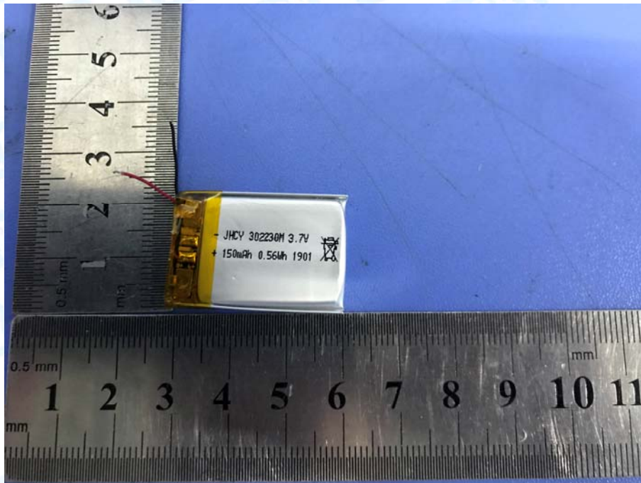
Photo 14 Battery Parameter Photo
