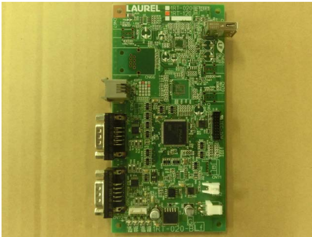
1RT-020-B(1RT-120) (Component Side)
