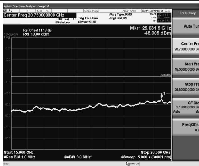
Band41_10MHz_QPSK_41190_1RB#0
