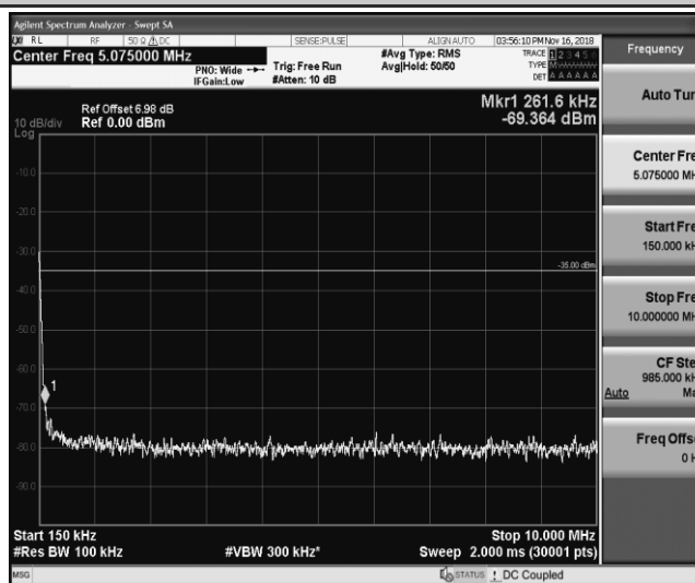
Band41_10MHz_QPSK_41190_1RB#0
