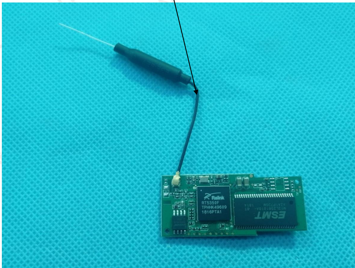
ANTENNA
