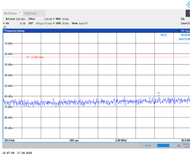
Band26-10MHz-QPSK-26740-1RB#0-Range2:0.15~30MHz
