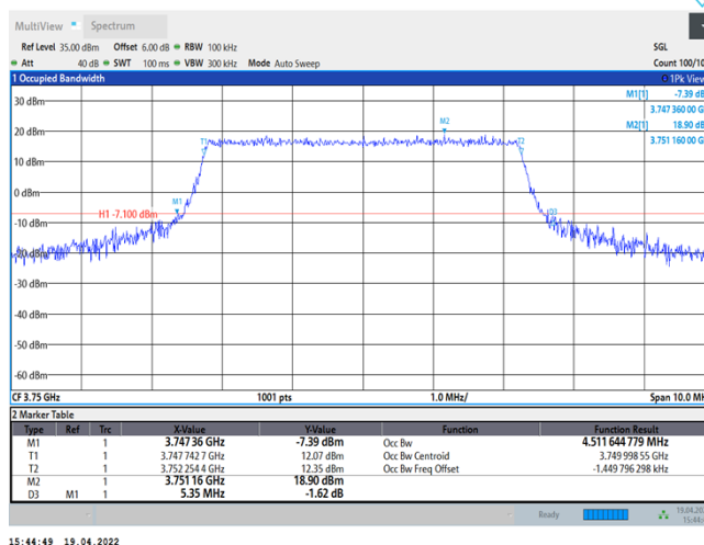
Band43-5MHz-QPSK-45090-25RB#0
