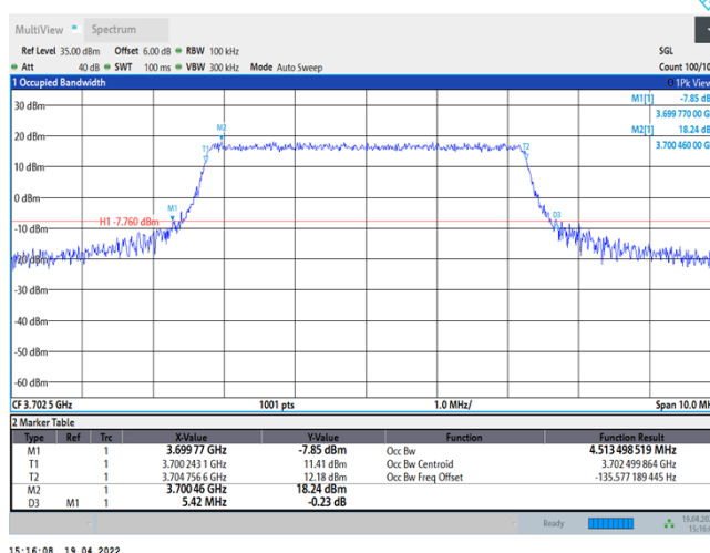
Band43-5MHz-QPSK-45090-25RB#0
