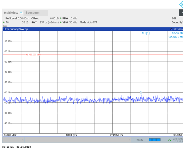
Band43-20MHz-QPSK-44690-1RB#0-Range2:0.15~30MHz
