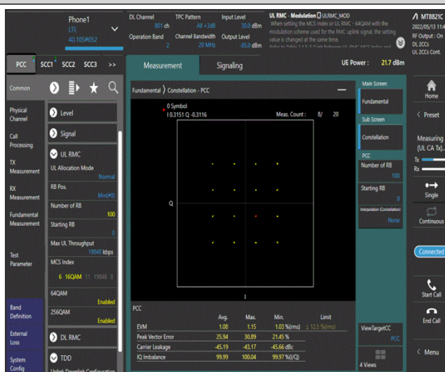
2-2-20MHz-20MHz-16QAM-16QAM-18801-18999-100RB#0-100RB#0
