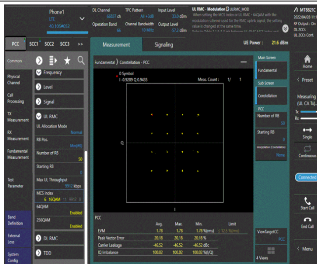
66-66-10MHz-10MHz-16QAM-16QAM-132373-132472-50RB#0-50RB#0
