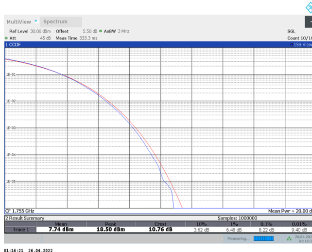
66-66-20MHz-20MHz-QPSK-QPSK-132323-132521-100RB#0-100RB#0
