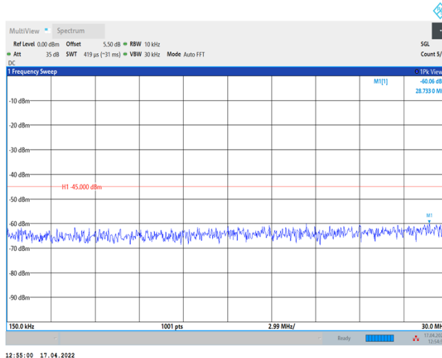
Band7-20MHz-QPSK-20850-1RB#0-Range2:0.15~30MHz
