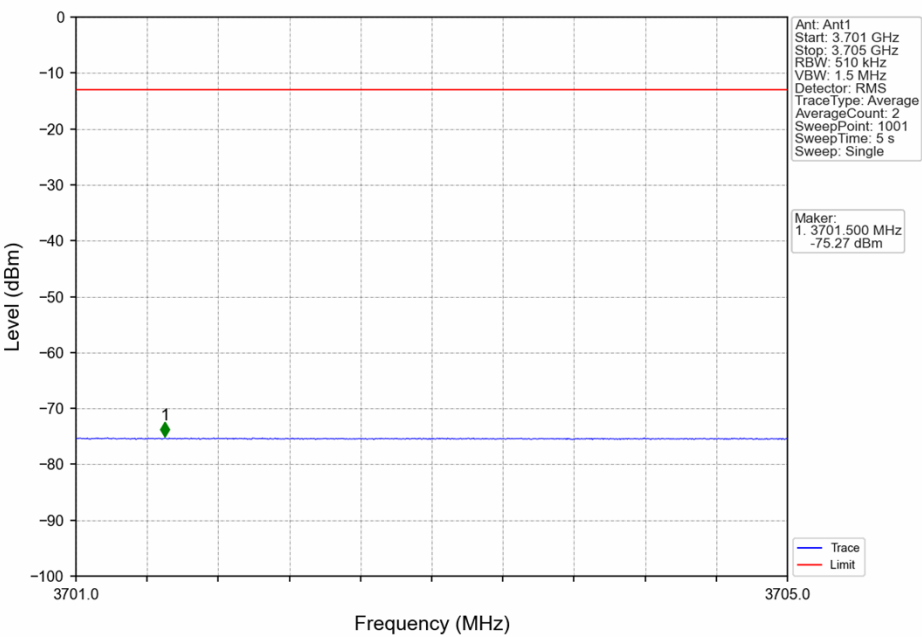
n48_30kHz_SISO_NTNV_20MHz_CP-OFDM QPSK_3690MHz_Inner_1RB_Right
