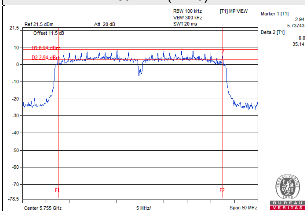
802.11n (HT40)
