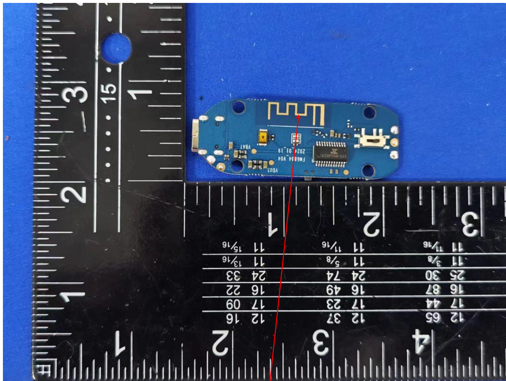
PCB ANT
