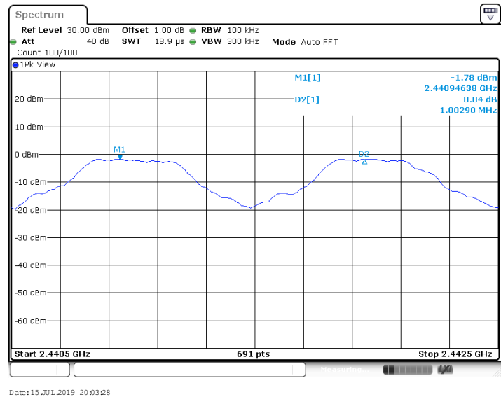
\pi/4 -DQPSK Modulation
