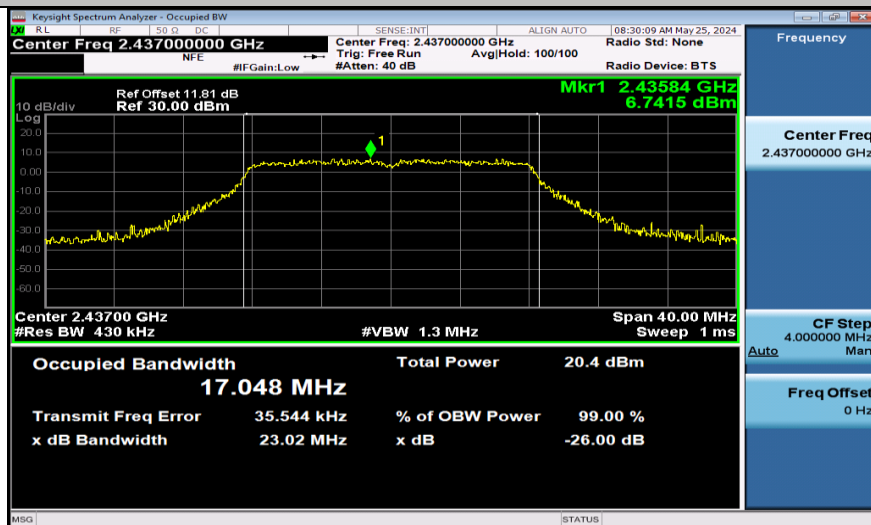
11G-Ant1-2437
