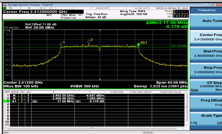
11N20ISO-Ant1-2412-PASS
