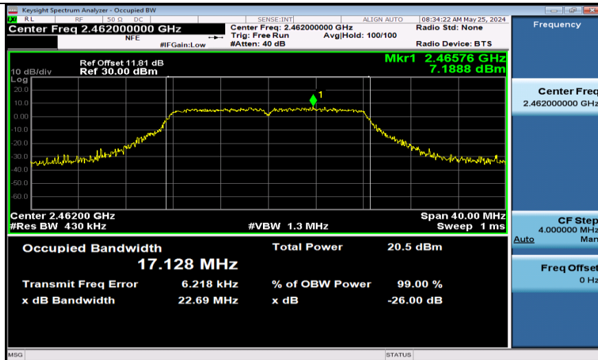
11G-Ant1-2462
