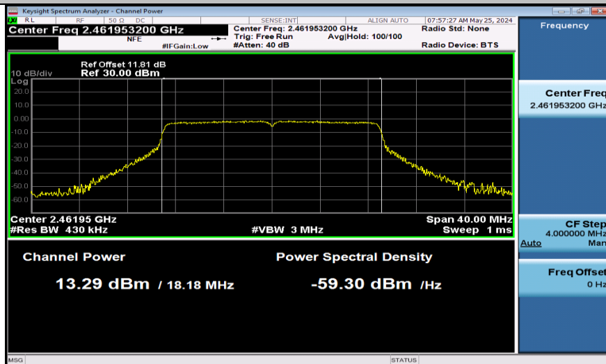
11N20ISO-Ant1-2462-PASS
