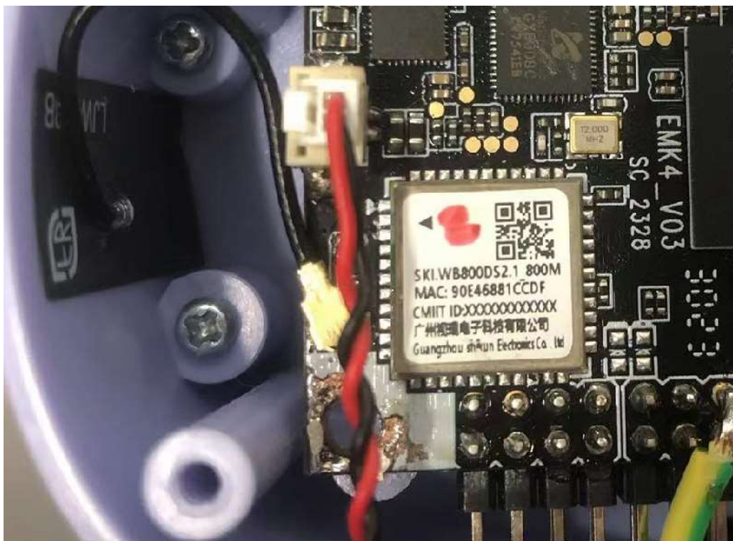
WiFi module
