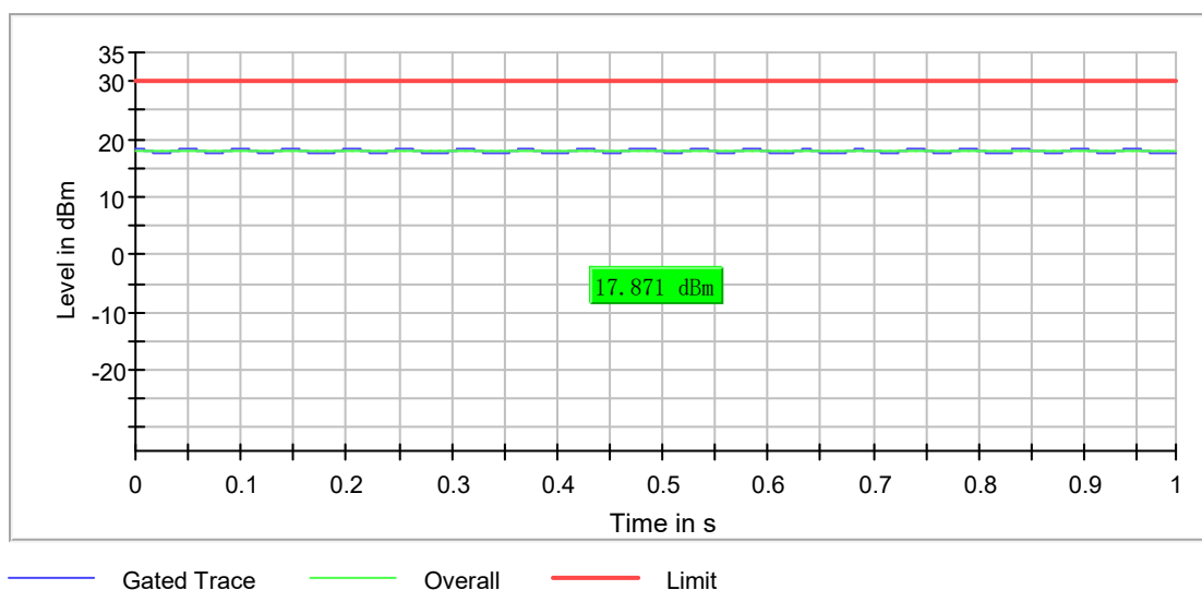
Data of IEEE 802.11 b
