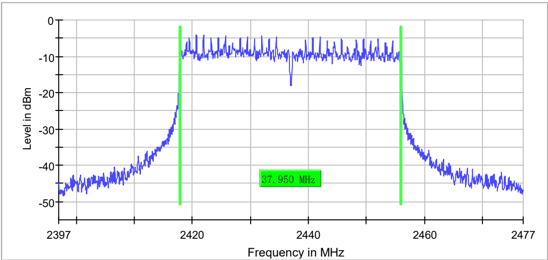
Mode 1 / CH5 (2437MHz)
