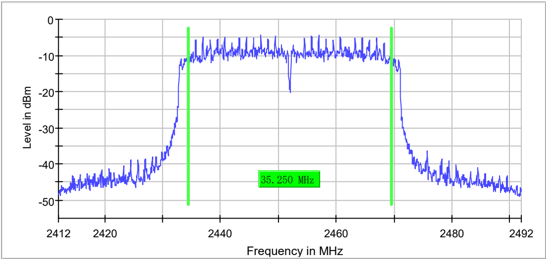
Mode 1 / CH8 (2452MHz)
