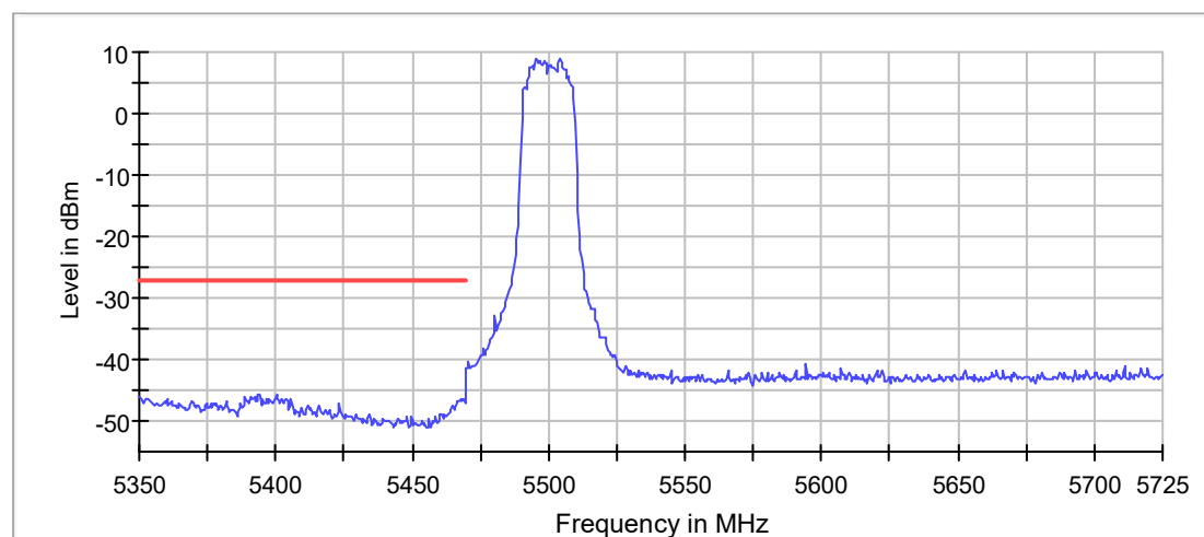
Band Edge
