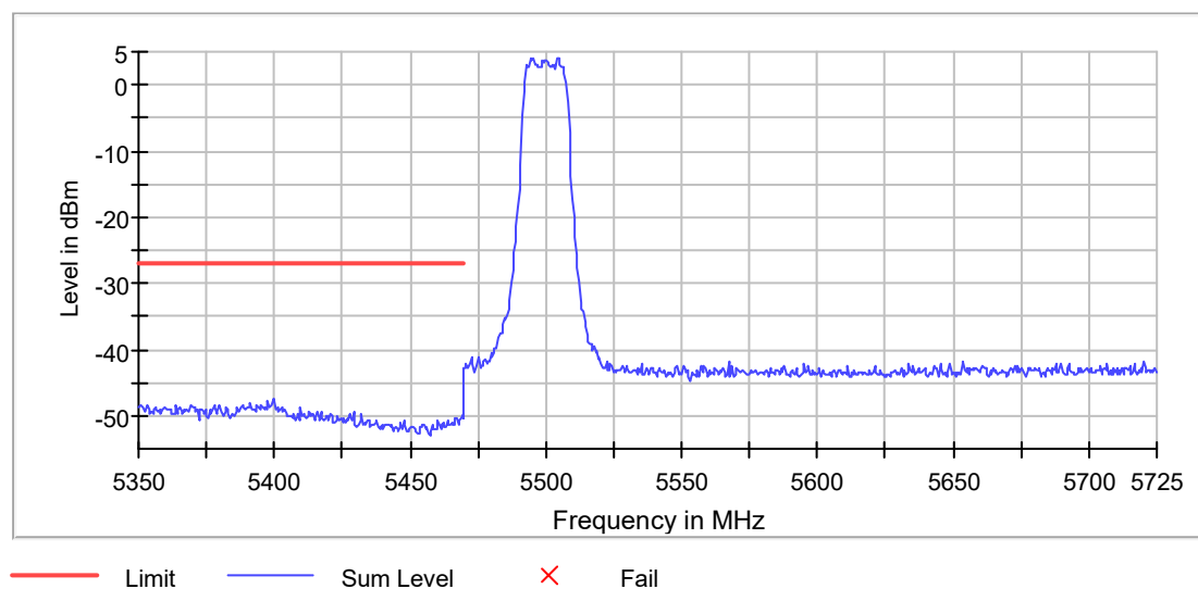
Band Edge
