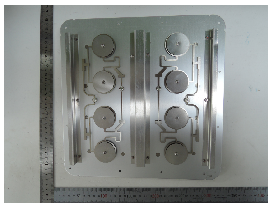
<LTE Antenna>
