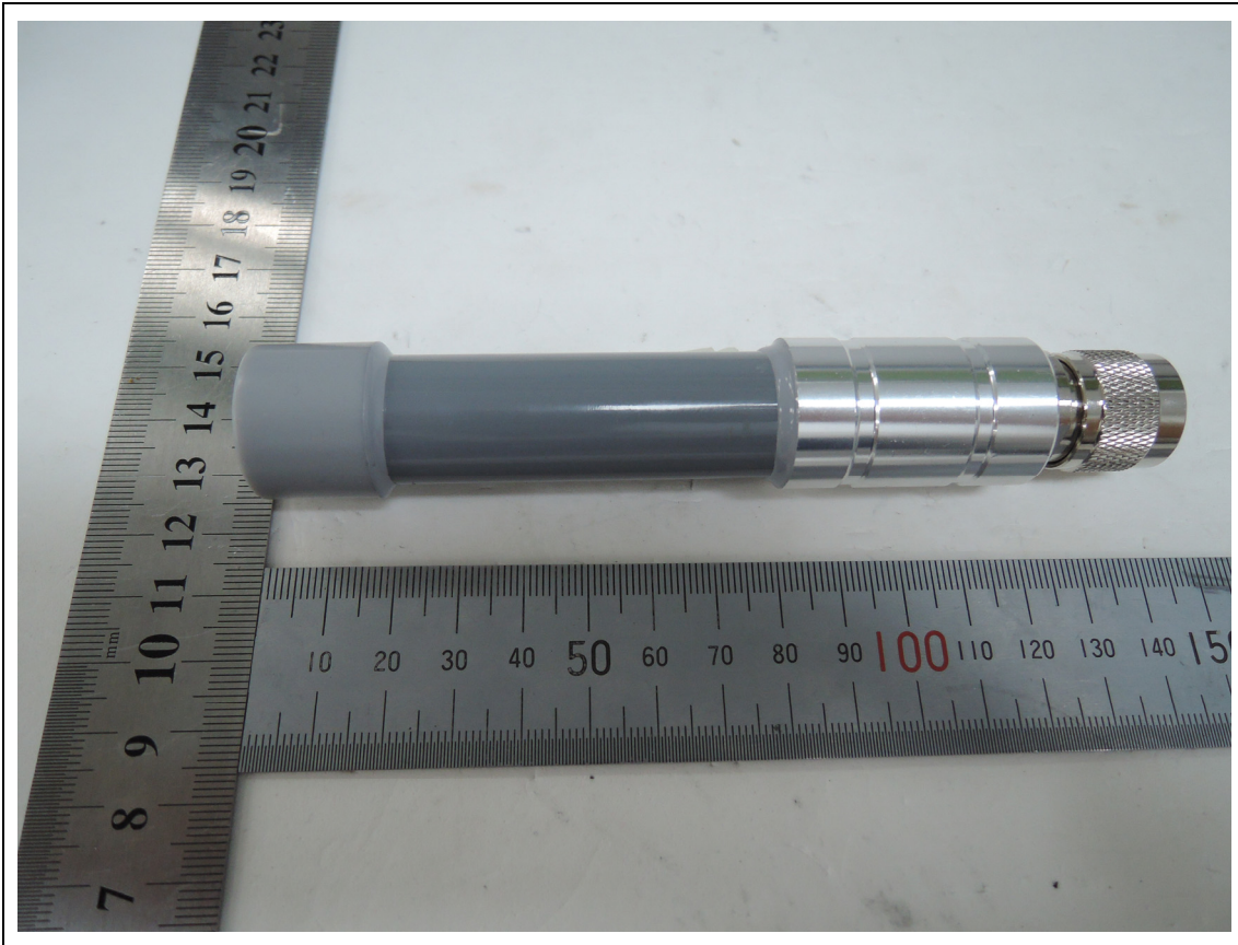
<GPS Antenna>
