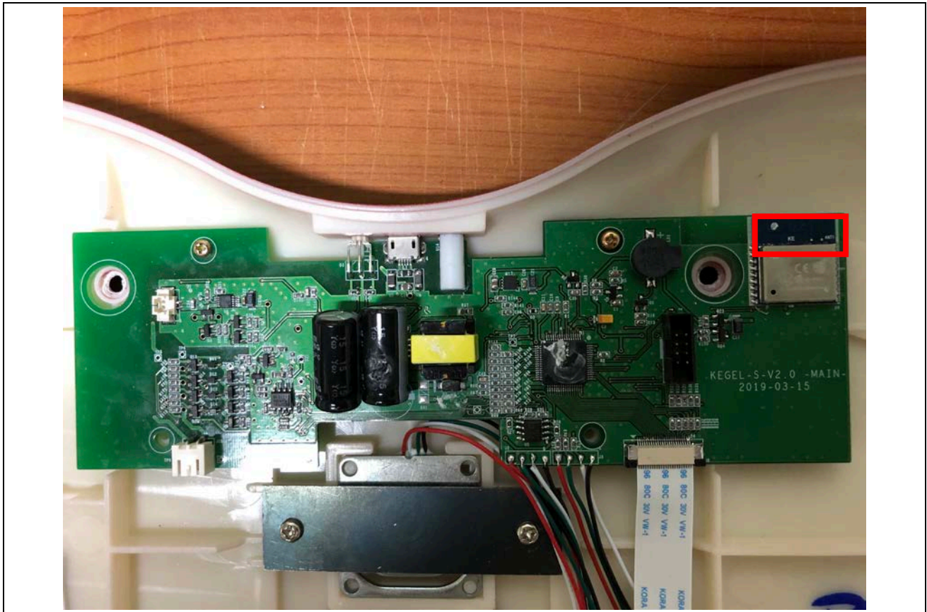
Antenna-Add Antenna
