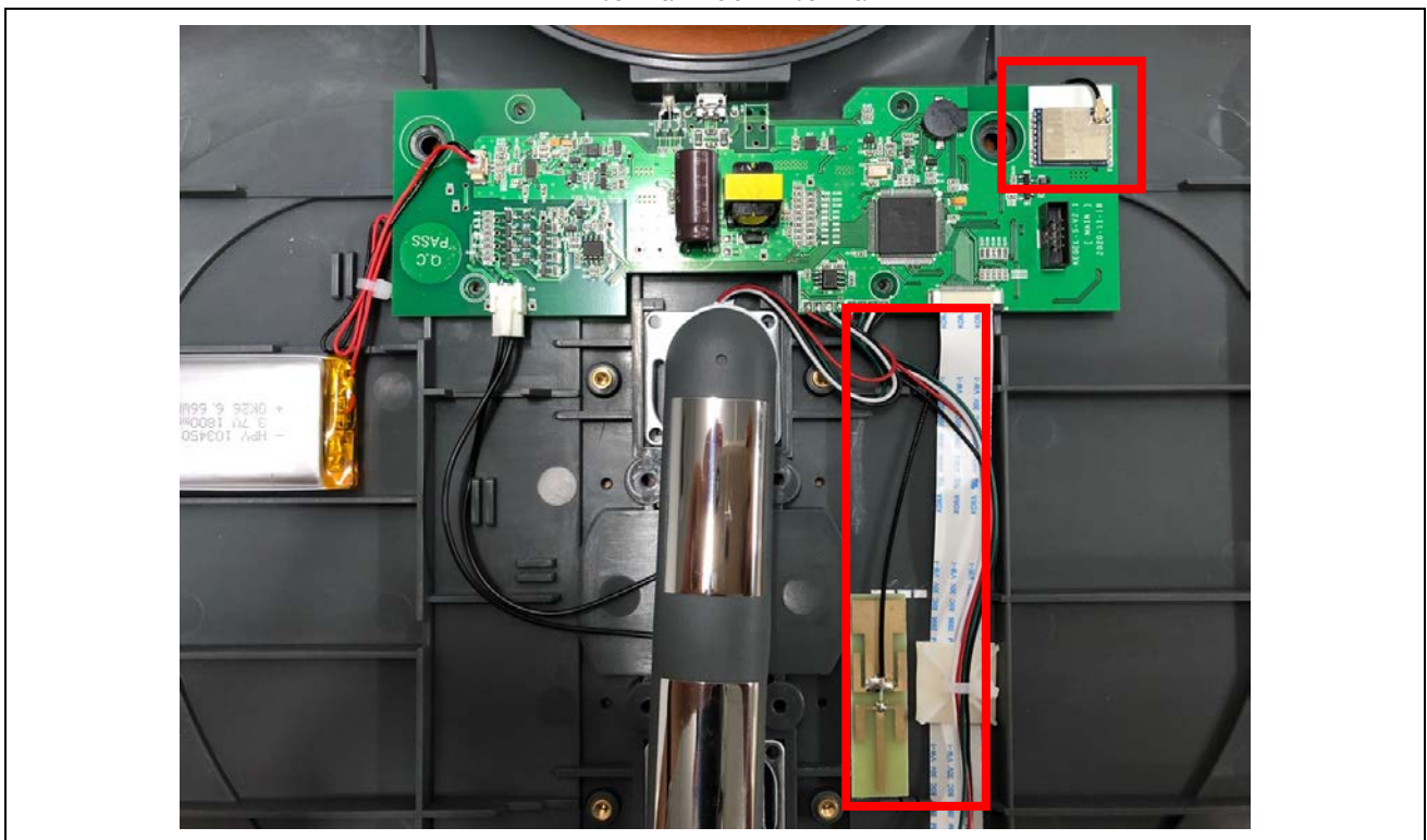
Antenna-Add Antenna
