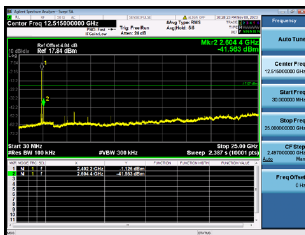
GFSK 2402MHz
