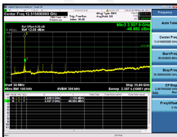
GFSK 2440MHz
