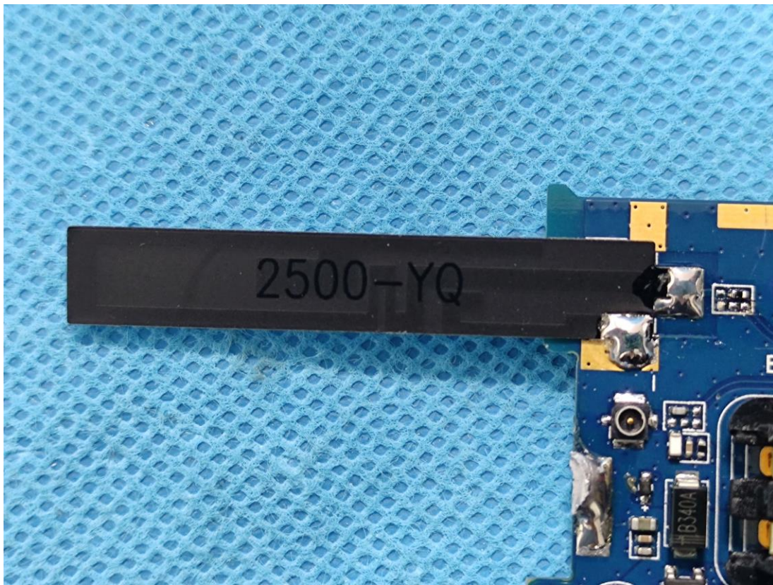
WWAN Antenna
