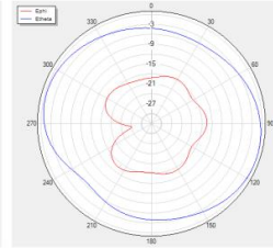
Theta=90 freq=2500MHz
