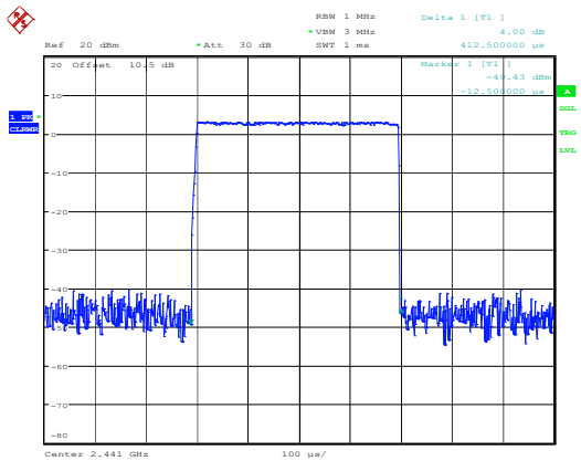
DH1_Hopping
