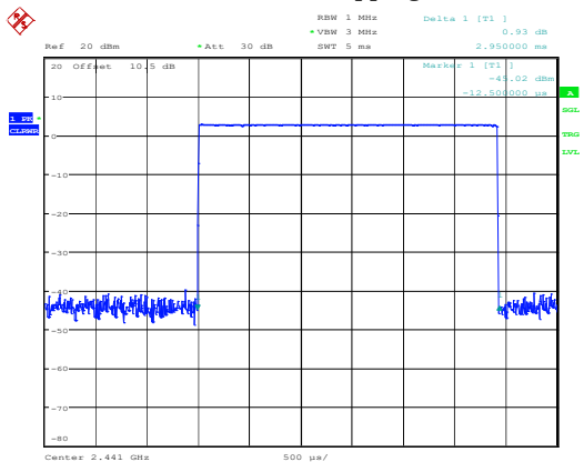
DH5_Hopping
