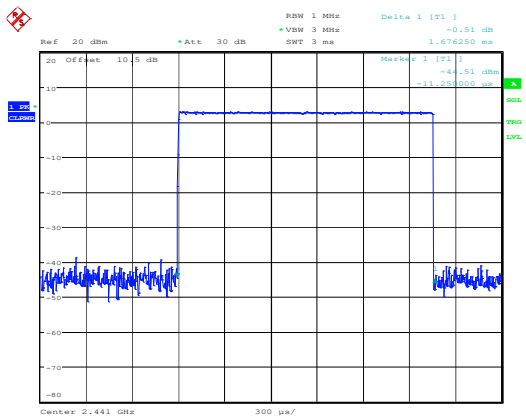
DH3_Hopping
