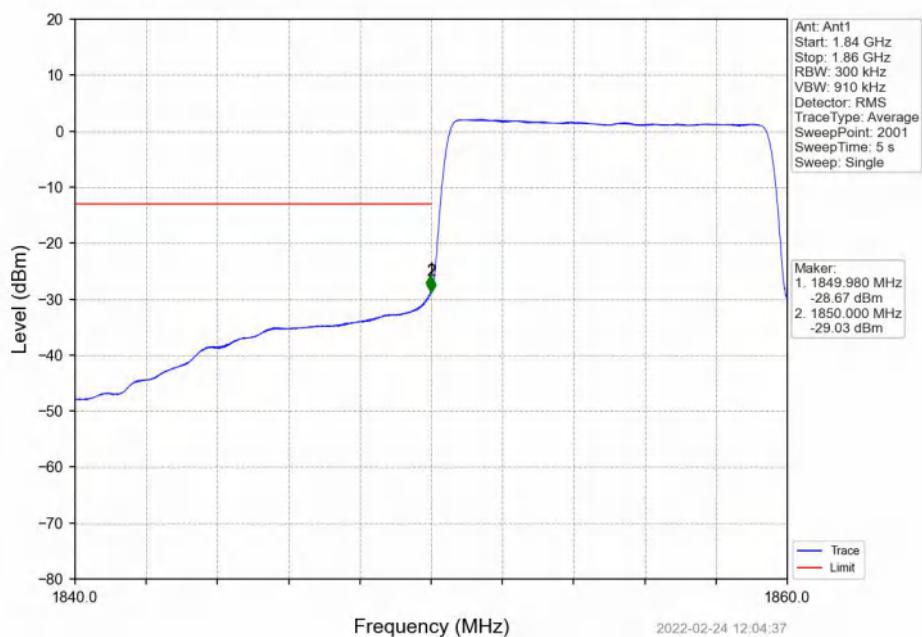
Band2_10MHz_QPSK_LCH_1855MHz_RB_50_0_NTNV
