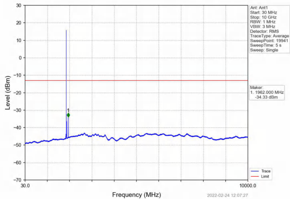
Band2_10MHz_16QAM_MCH_1880MHz_RB_1_0_NTNV
