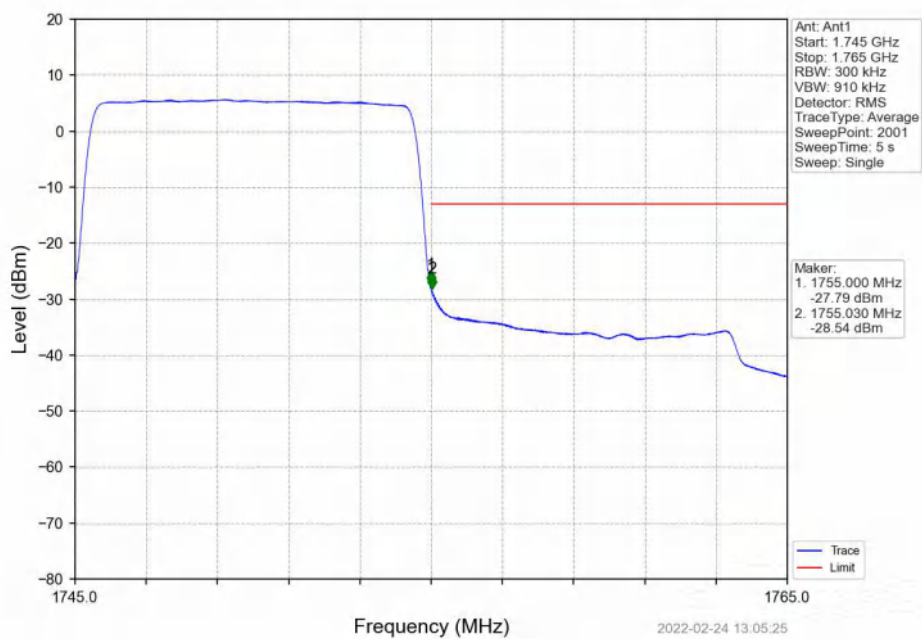
Band4_10MHz_QPSK_HCH_1750MHz_RB_50_0_NTNV
