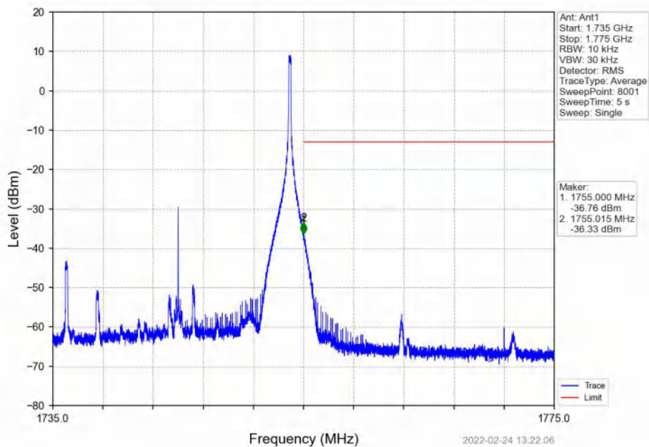
Band4_20MHz_QPSK_HCH_1745MHz_RB_100_0_NTNV
