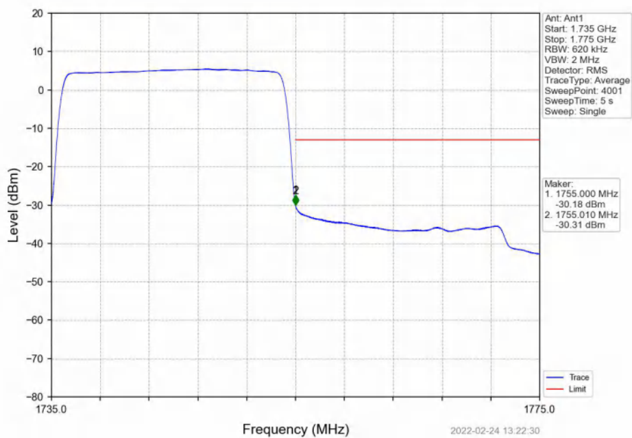
Band4_20MHz_QPSK_HCH_1745MHz_RB_100_0_NTNV
