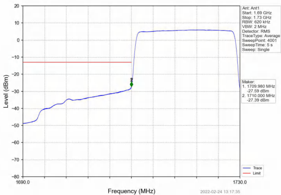
Band4_20MHz_QPSK_LCH_1720MHz_RB_100_0_NTNV
