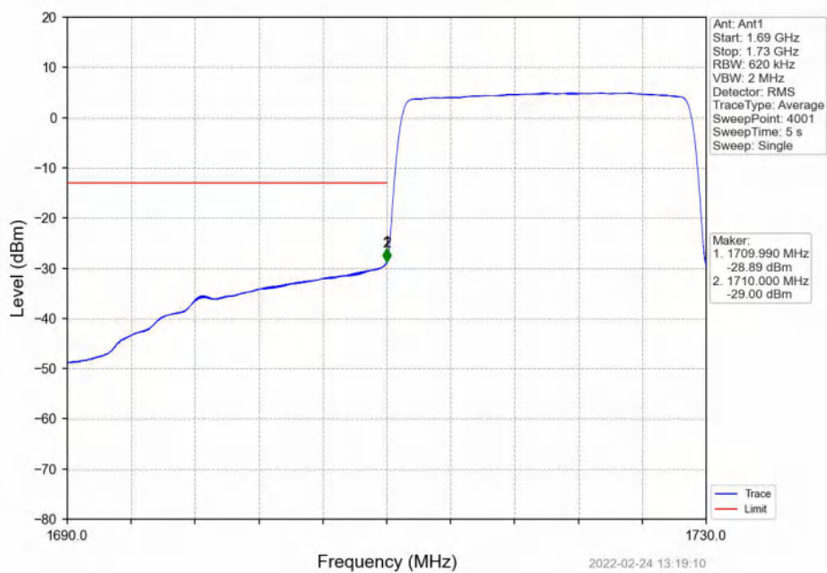
Band4_20MHz_16QAM_LCH_1720MHz_RB_100_0_NTNV
