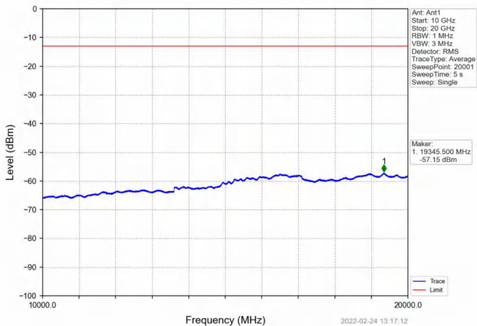
Band4_20MHz_QPSK_LCH_1720MHz_RB_100_0_NTNV
