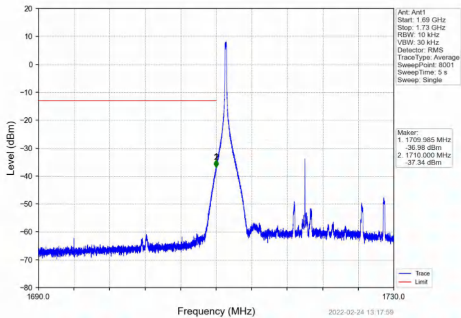
Band4_20MHz_16QAM_LCH_1720MHz_RB_1_0_NTNV
