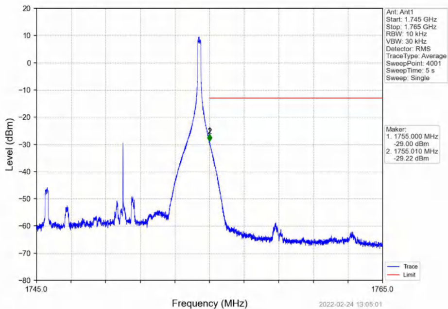
Band4_10MHz_QPSK_HCH_1750MHz_RB_50_0_NTNV
