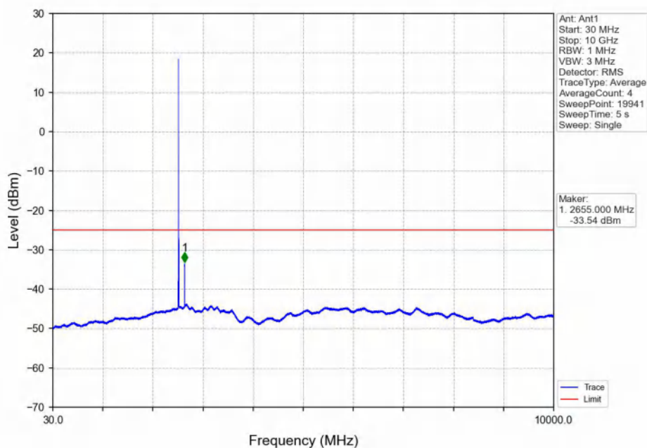
Band7_5MHz_QPSK_MCH_2535MHz_RB_1_0_NTNV
