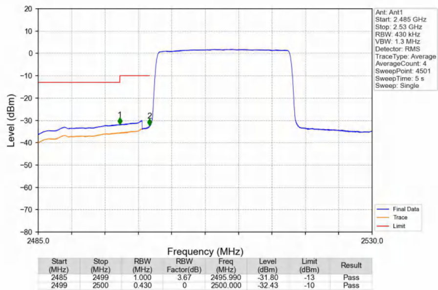
Band7_20MHz_QPSK_LCH_2510MHz_RB_100_0_NTNV
