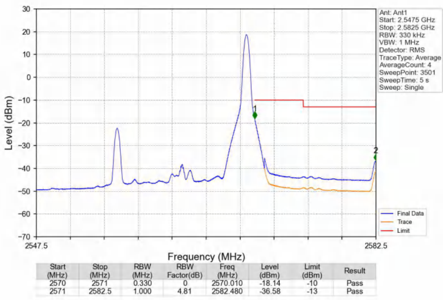
Band7_15MHz_QPSK_HCH_2562.5MHz_RB_1_74_NTNV
