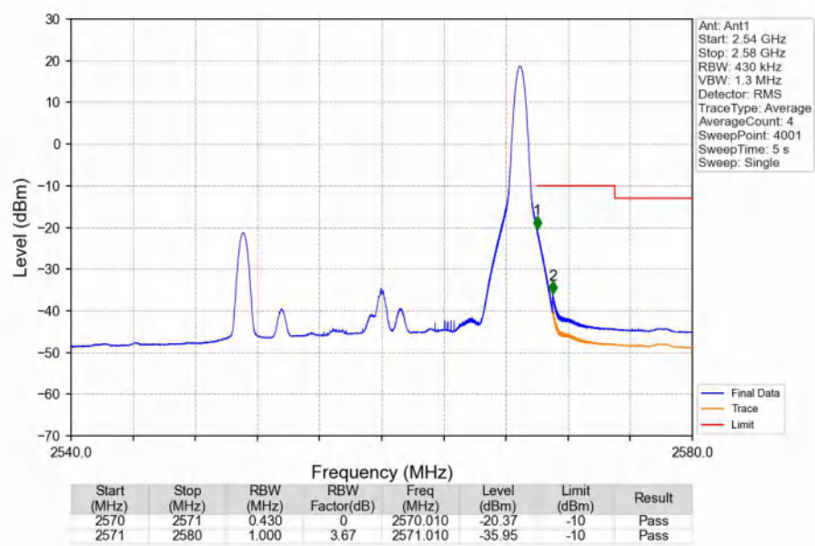
Band7_20MHz_QPSK_HCH_2560MHz_RB_1_99_NTNV
