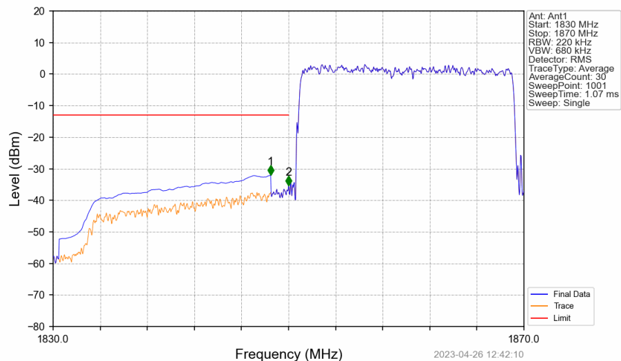
Band2 20MHz QPSK LCH 1860MHz RB 100 0 NTN
