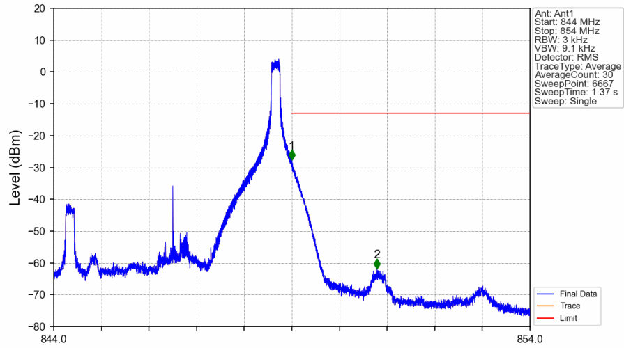
Band5 5MHz 16QAM HCH 846.5MHz RB 1 24 NTV
