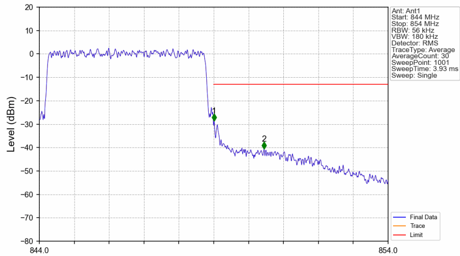
Band5 5MHz 16QAM HCH 846.5MHz RB 25 0 NTV
