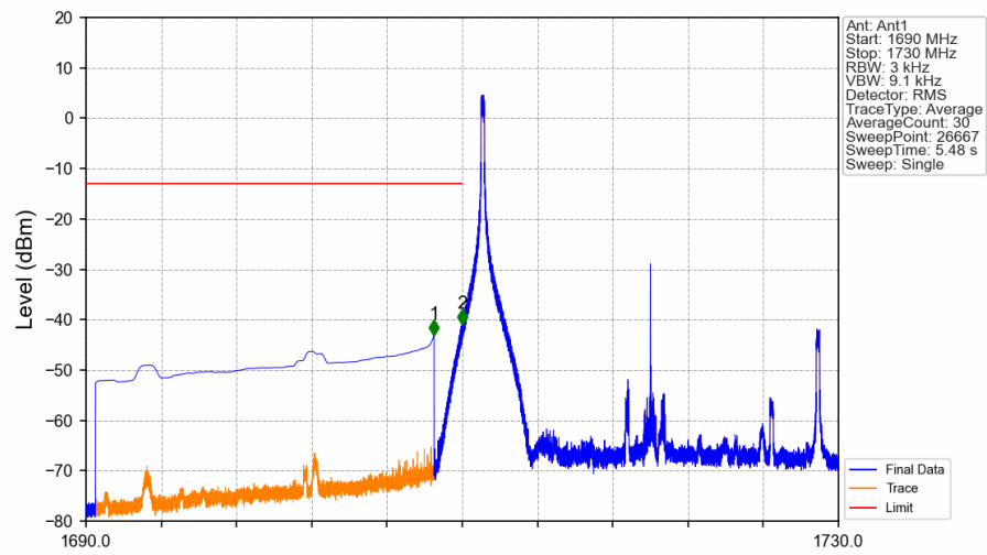
Band66_20MHz_16QAM_LCH_1720MHz_RB_1_0_NTNV
