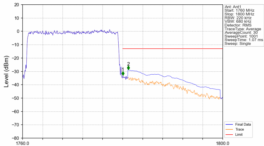
Band66 20MHz 16QAM HCH 1770MHz RB 100 0 NTNV
