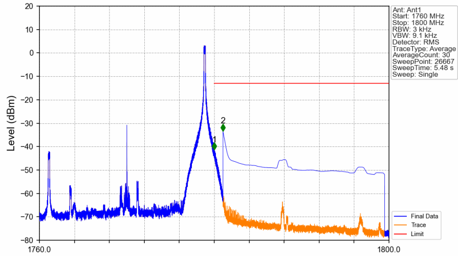
Band66 20MHz 16QAM HCH 1770MHz RB 1 99 NTNV
