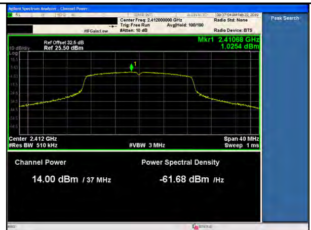
11n-20MHz-PWR-Low-MCS7
