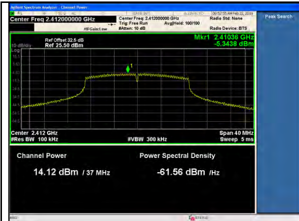
11n-20MHz-PSD-Low-MCS0
