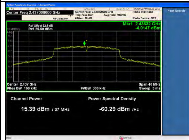
11n-20MHz-PSD-Mid-MCS0
