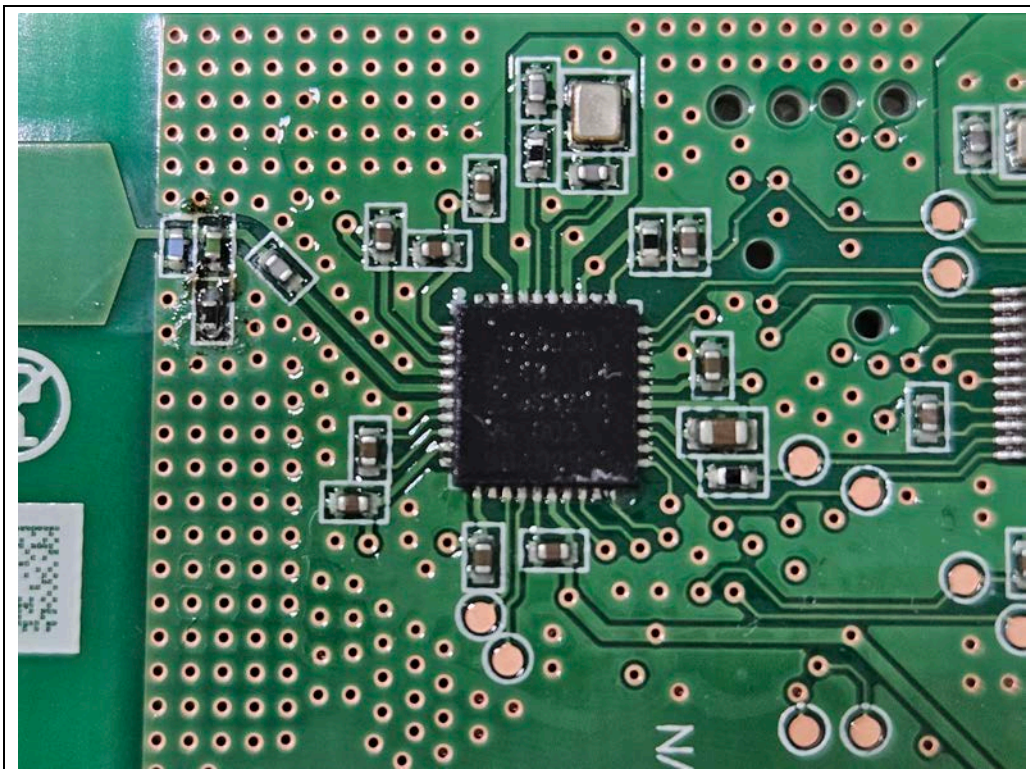
<UWB Module>
