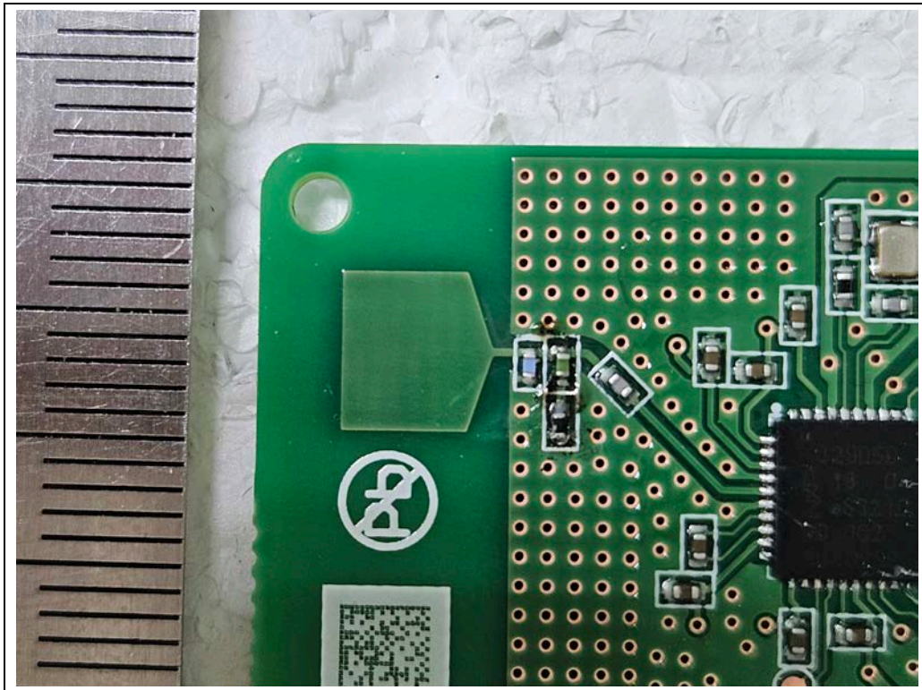
<UWB Antenna>
