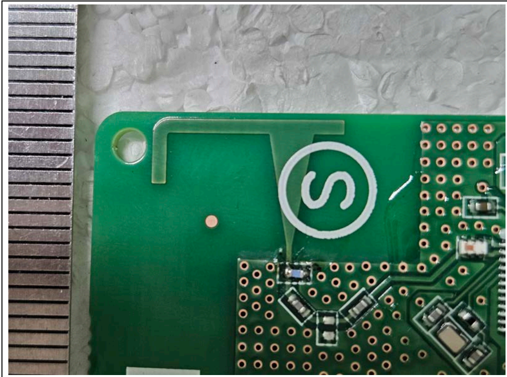
<BLE Antenna>
