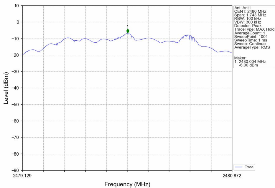
PSD NVNT BLE 2M 2480MHz Ant1
