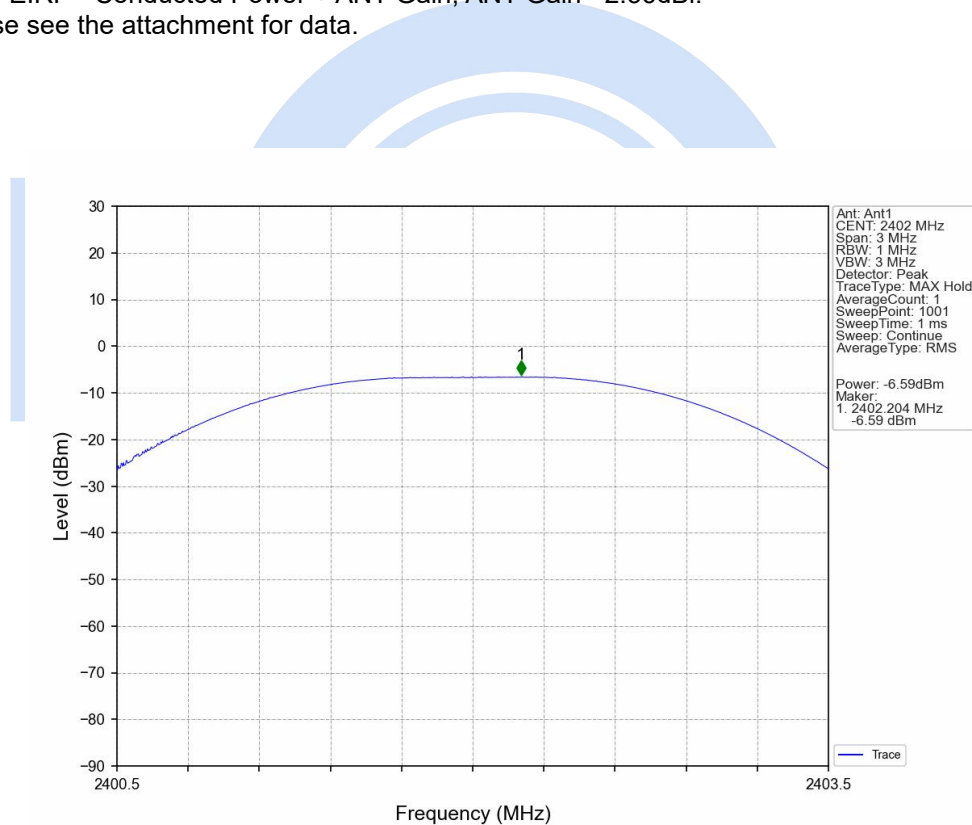
Peak Power NVNT BLE 1M 2402MHz Ant1
