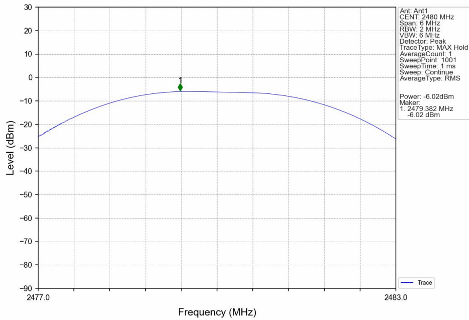
Peak Power NVNT BLE 2M 2480MHz Ant1
