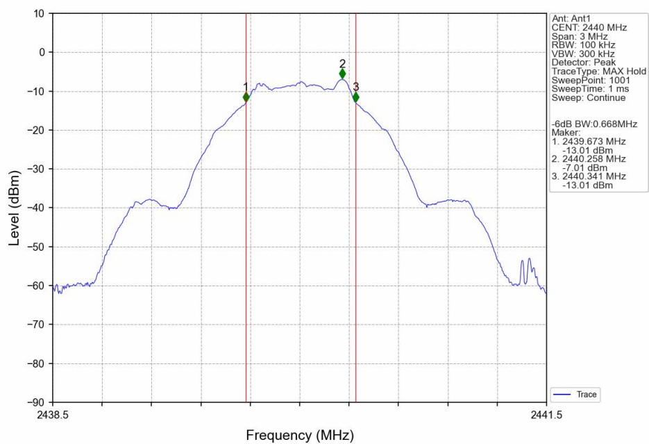
-6dB Bandwidth NVNT BLE 1M 2440MHz Ant1
