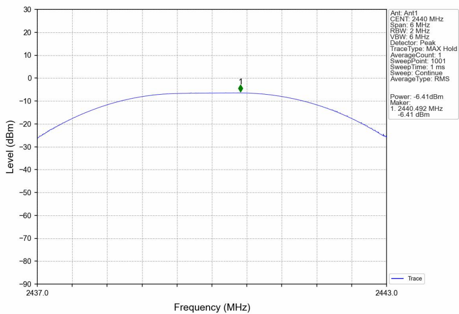
Peak Power NVNT BLE 2M 2440MHz Ant1
