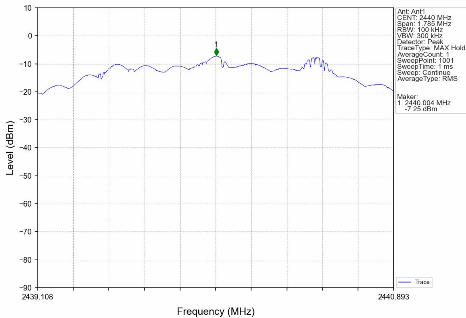
PSD NVNT BLE 2M 2440MHz Ant1
