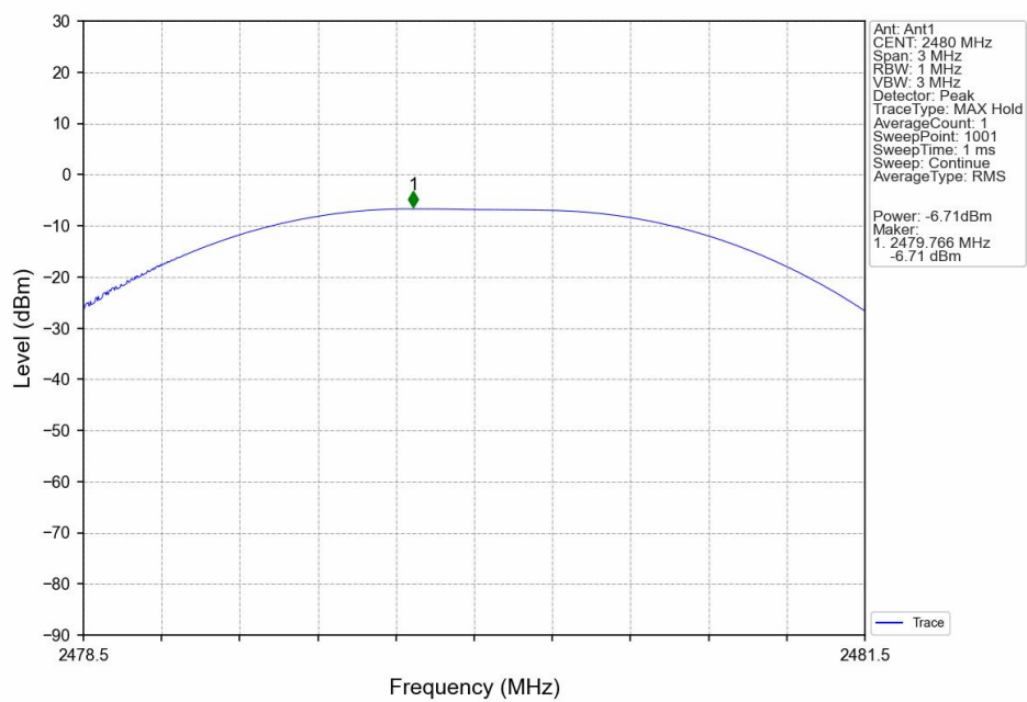
Peak Power NVNT BLE 1M 2480MHz Ant1
