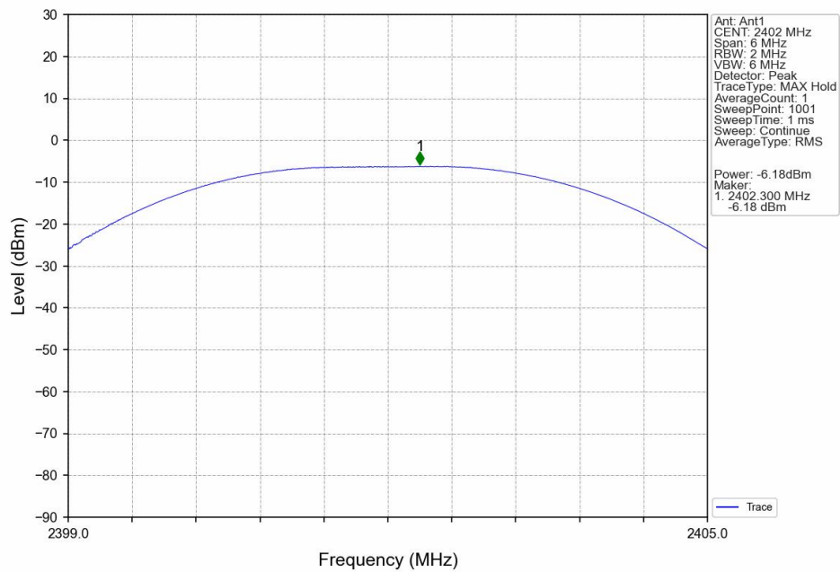
Peak Power NVNT BLE 2M 2402MHz Ant1
