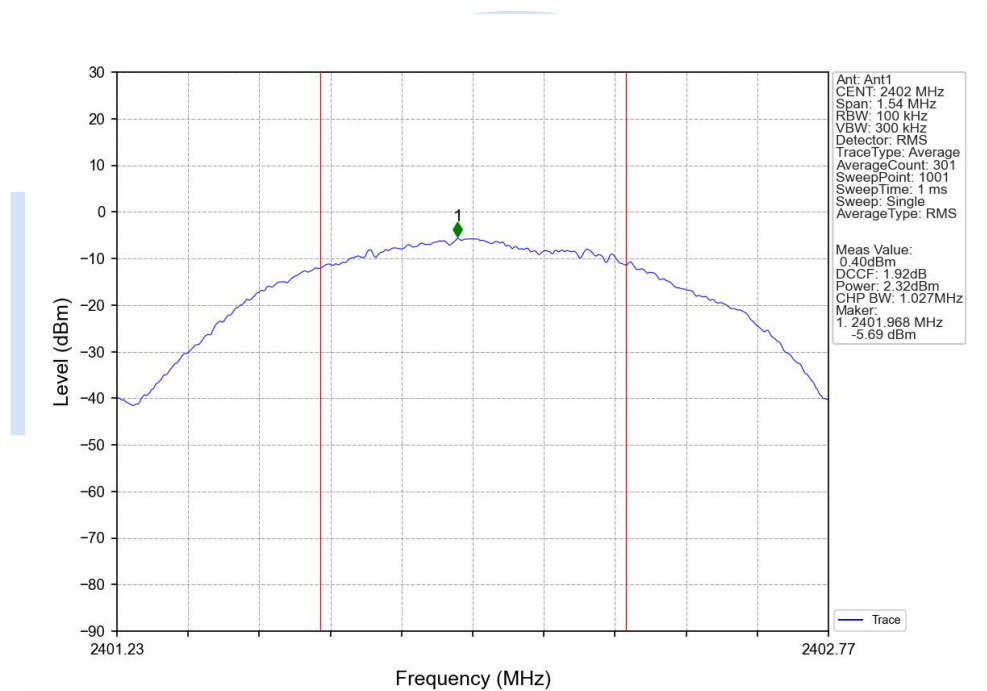
Peak Power NVNT BLE 1M 2402MHz Ant1
