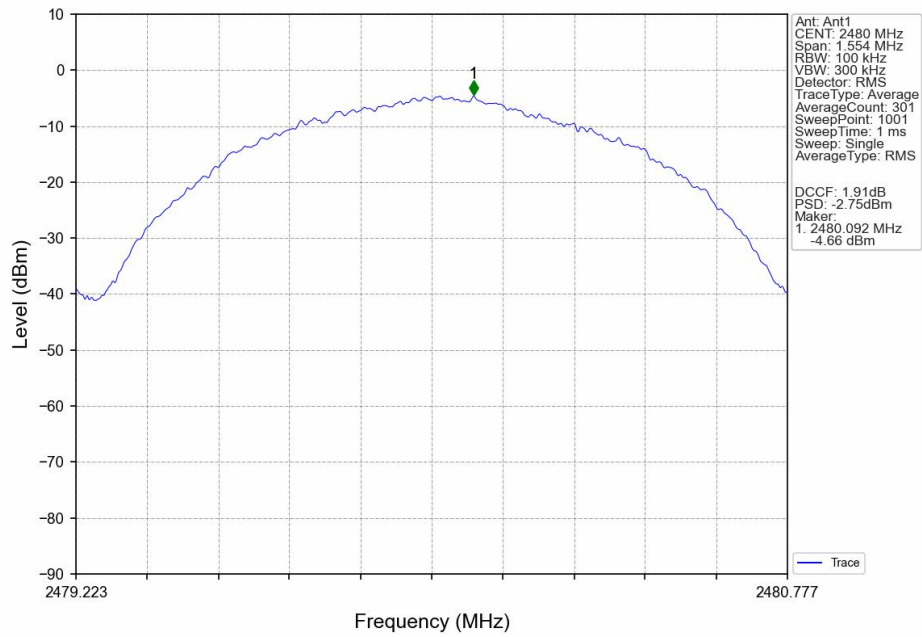
PSD NVNT BLE 1M 2480MHz Ant1
