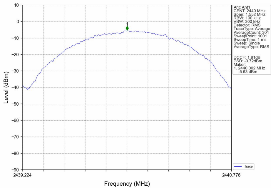
PSD NVNT BLE 1M 2440MHz Ant1
