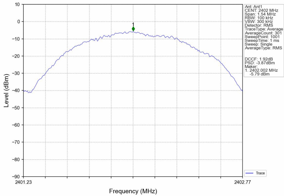
PSD NVNT BLE 1M 2402MHz Ant1
