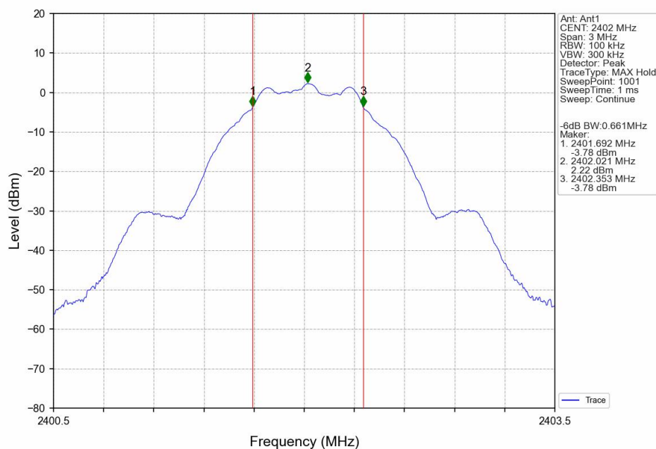
-6dB Bandwidth NVNT BLE 1M 2402MHz Ant1
