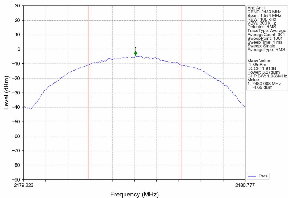
Peak Power NVNT BLE 1M 2480MHz Ant1
