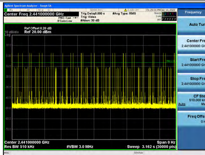
3DH3_Ant1_Hop
