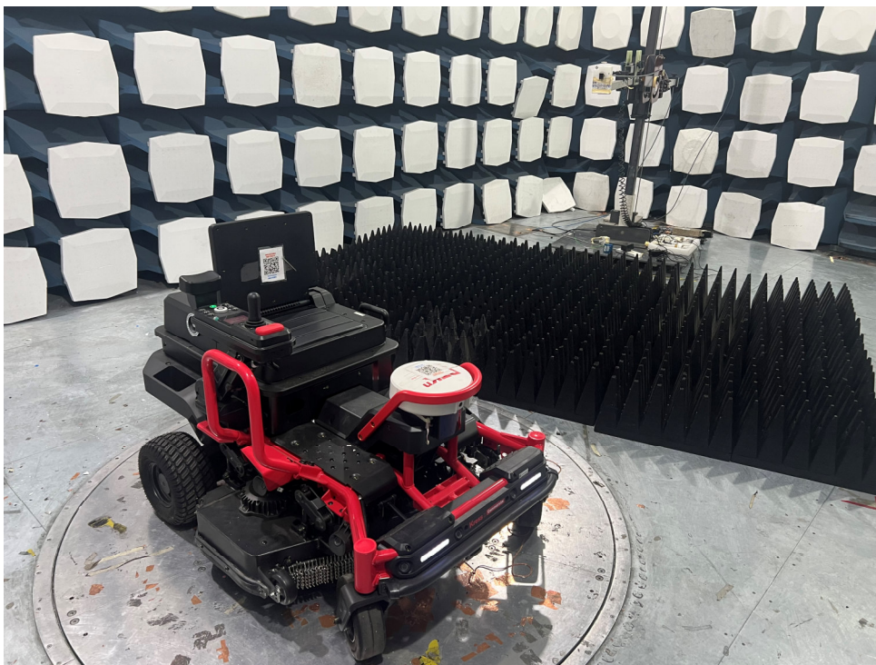
18GHz - 26.5GHz
