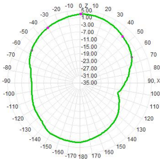
E1面-PHI=0
