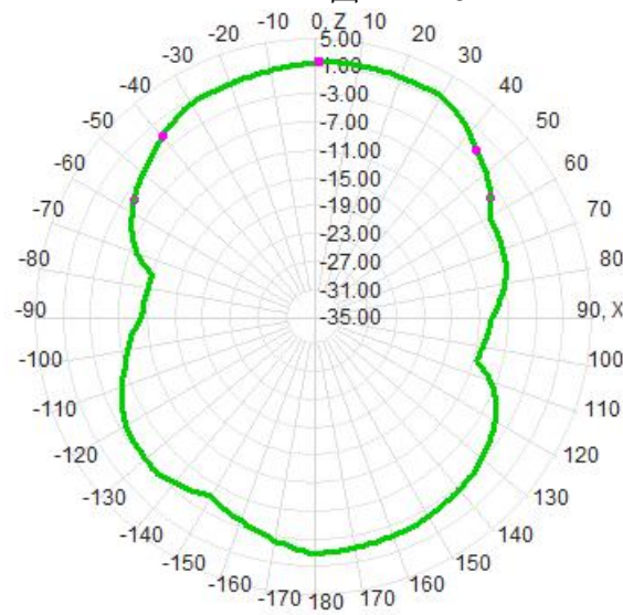
E1面-PHI=0
