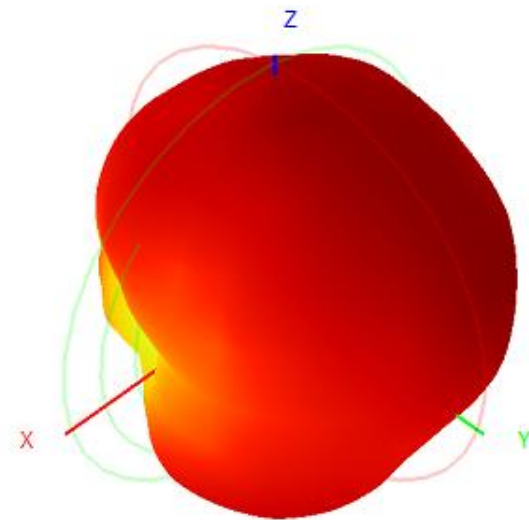
E1面-PHI=0
