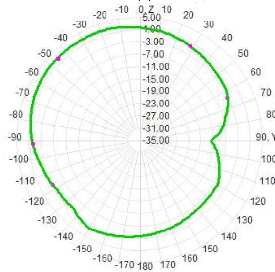
E2面-PHI=90
