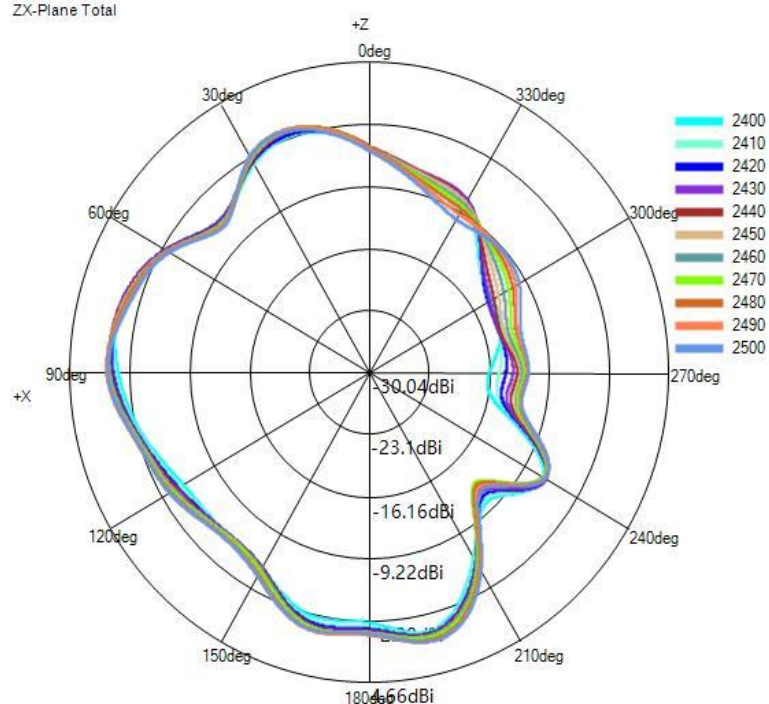
ZX-Plane Total
