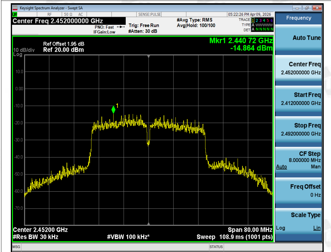
PSD NVNT ax40 2452MHz Ant1
