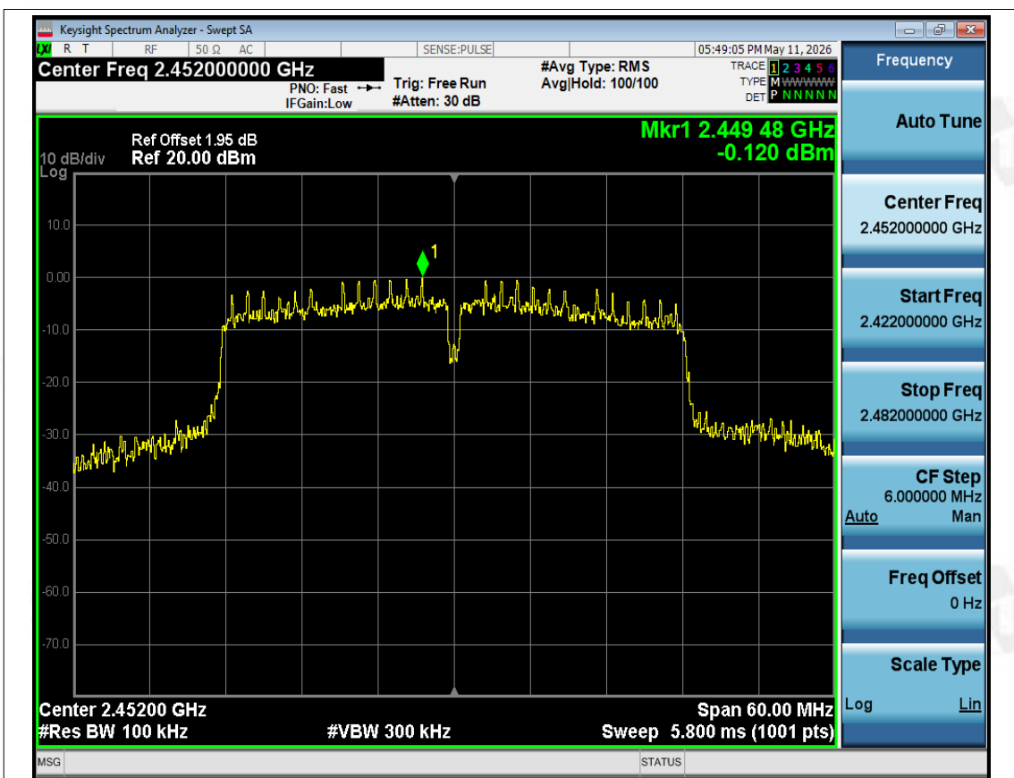
Band Edge NVNT ax40 2452MHz Ant1 Ref
