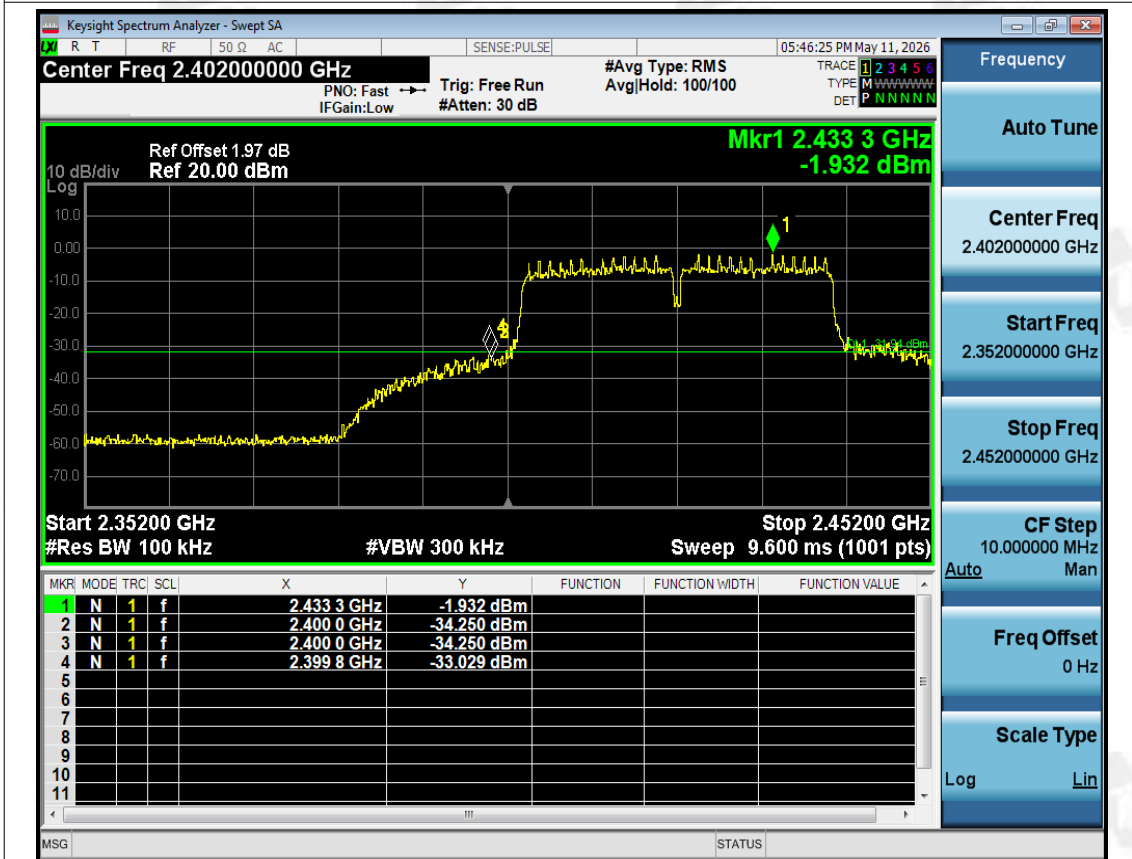
Band Edge NVNT ax40 2422MHz Ant1 Emission
