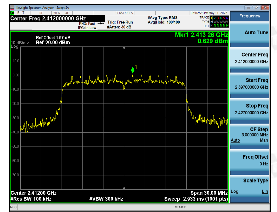
Band Edge NVNT ax20 2412MHz Ant1 Ref
