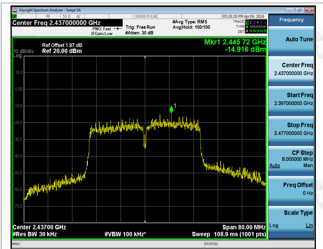
PSD NVNT ax40 2437MHz Ant1
