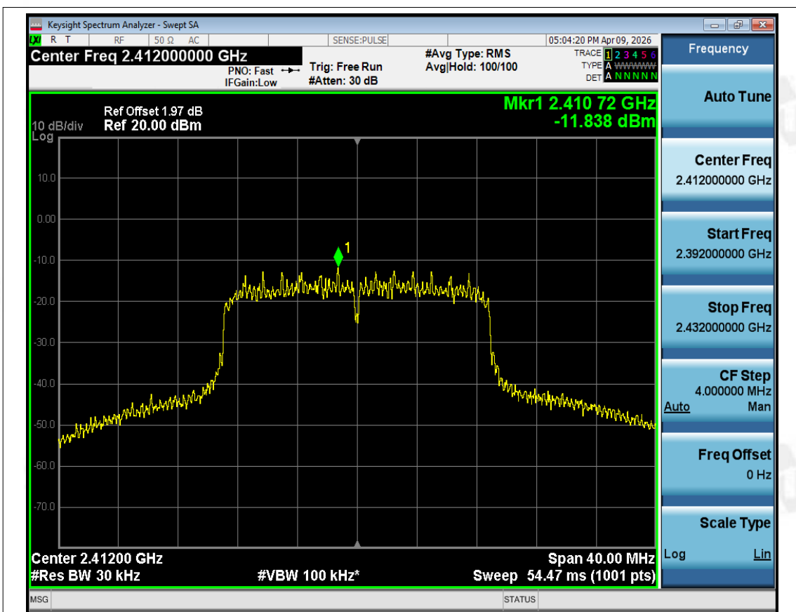
PSD NVNT ax20 2412MHz Ant1
