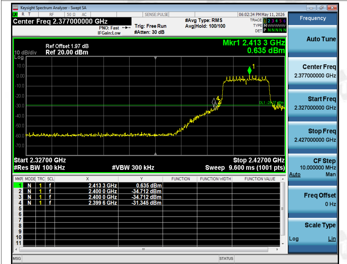
Band Edge NVNT ax20 2412MHz Ant1 Emission
