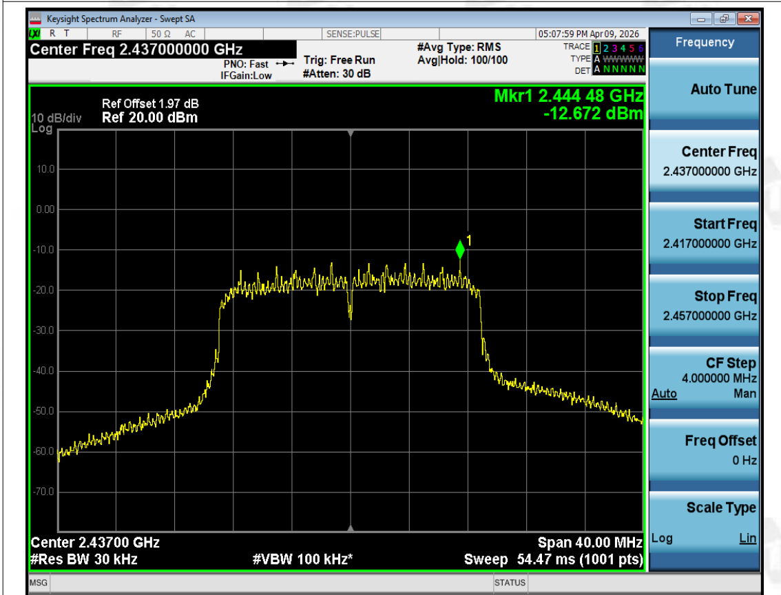
PSD NVNT ax20 2437MHz Ant1
