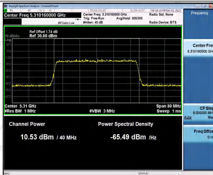
11AX40ISO_Ant1_5310
