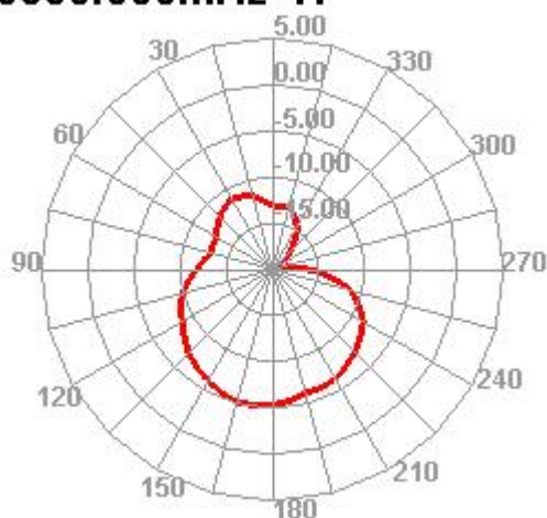
5850.000MHz H
