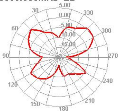
5850.000MHz E2
