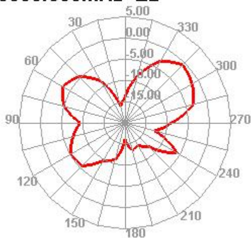
5500.000MHz E2
