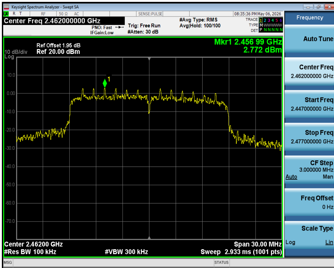
Band Edge NVNT ax20 2462MHz Ant1 Ref
