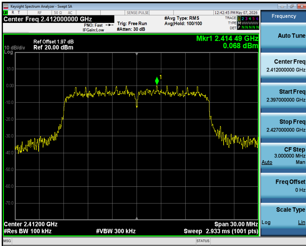
Band Edge NVNT ax20 2412MHz Ant1 Ref
