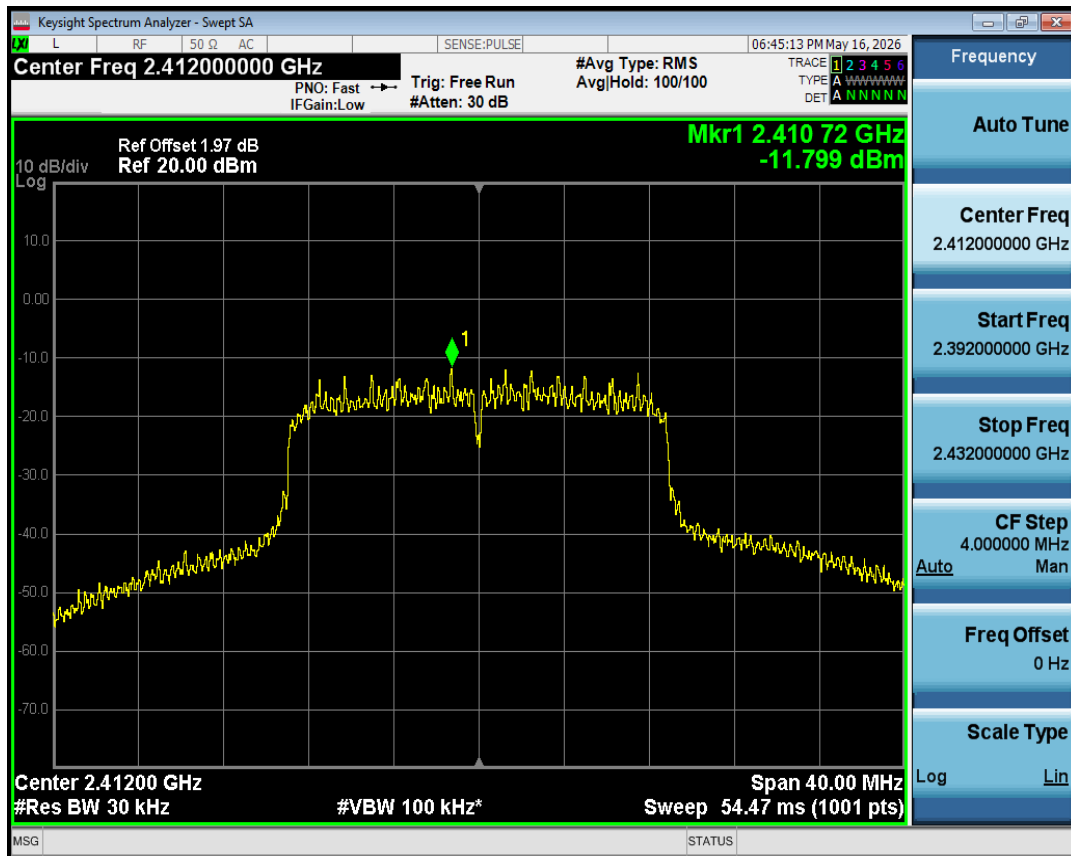
PSD NVNT ax20 2412MHz Ant1
