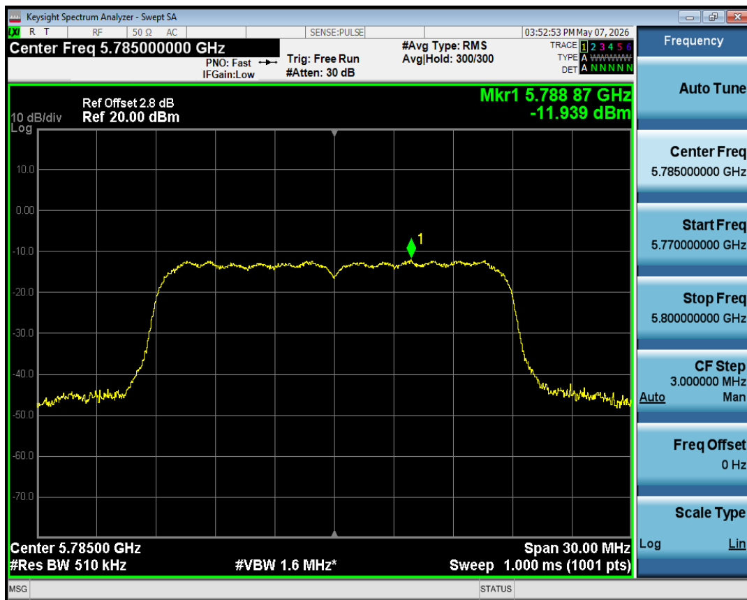
PSD NVNT ax20 5785MHz Ant1
